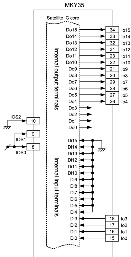
Fig. 3.8 IO Mode 4
