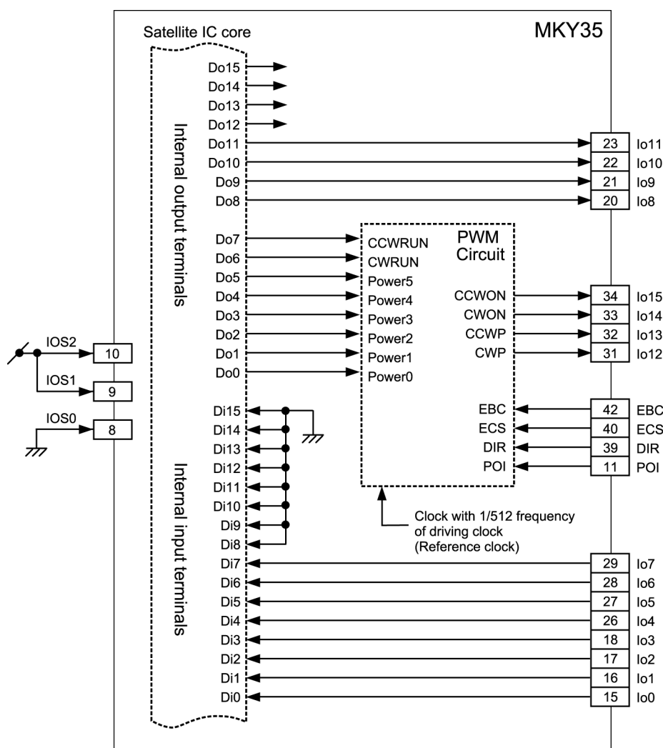
Fig. 4.9 PWM Mode 1
