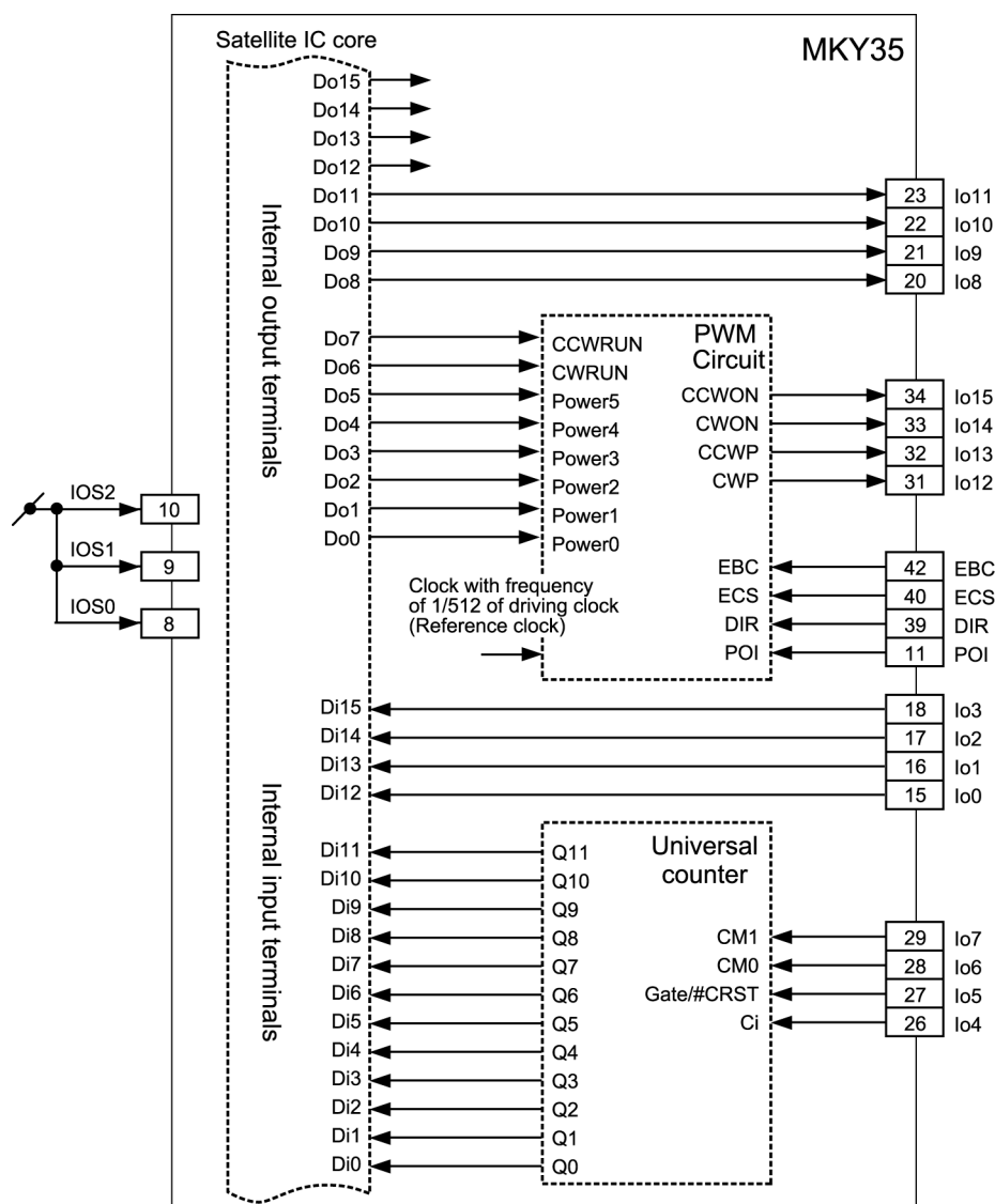
Fig. 4.14 PWM Mode 2
