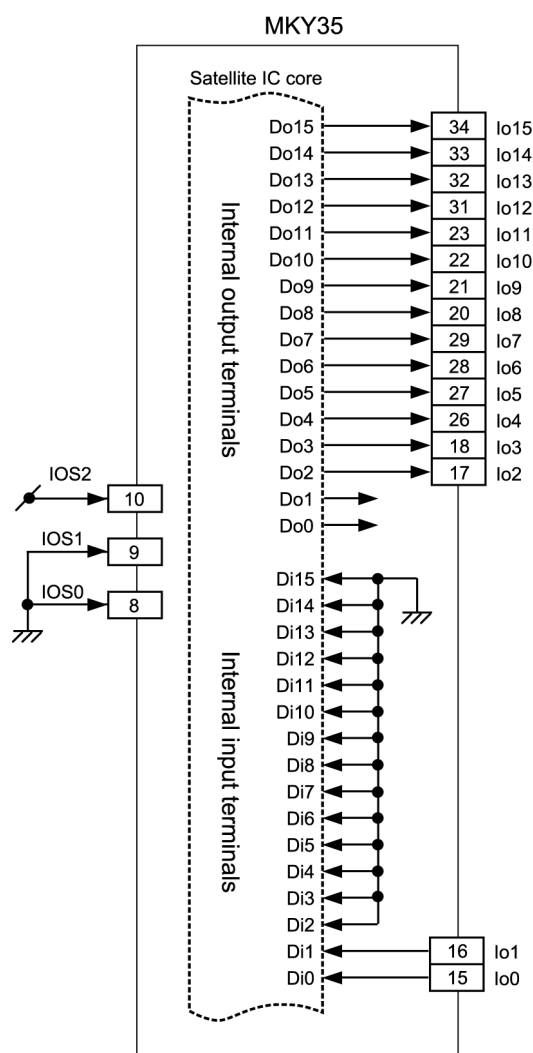
Fig.3.9 I/O Mode 5
