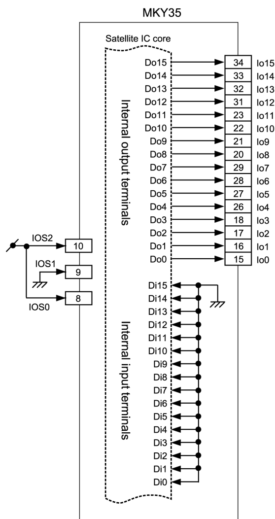
Fig.3.10 I/O Mode 6
