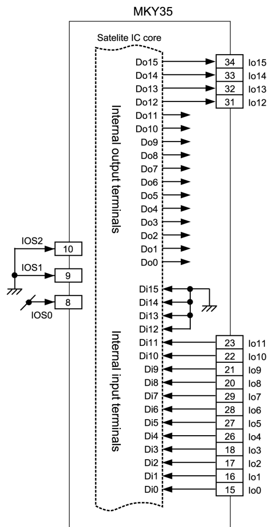
Fig. 3.6 I/O Mode 2
