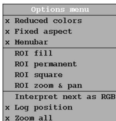
Figure 4.7: Options menu.
