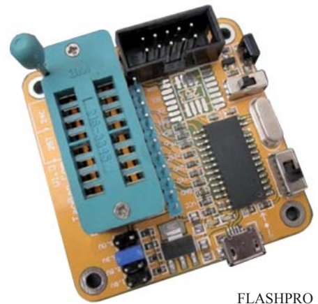
FLASHPRO programmer
