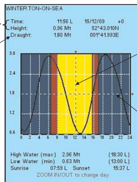
Fig. 3.9.2b - Tide Graph
