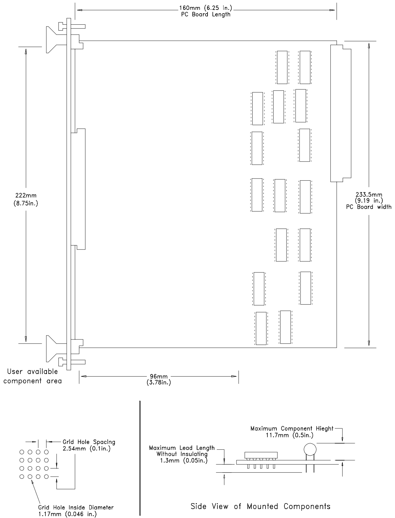
Figure 2-2. HP E1399A Dimensions
