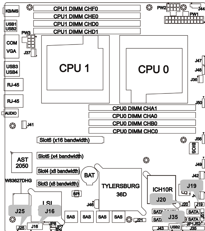
J16: Com2 Header
