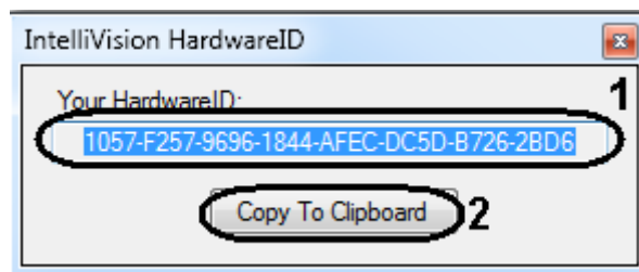
Fig. 6.3—1 HardwareID.exe utility
