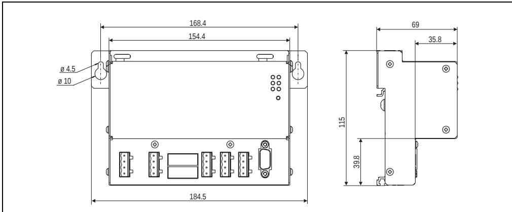
Figure 3: Dimensions 9A0100.11
