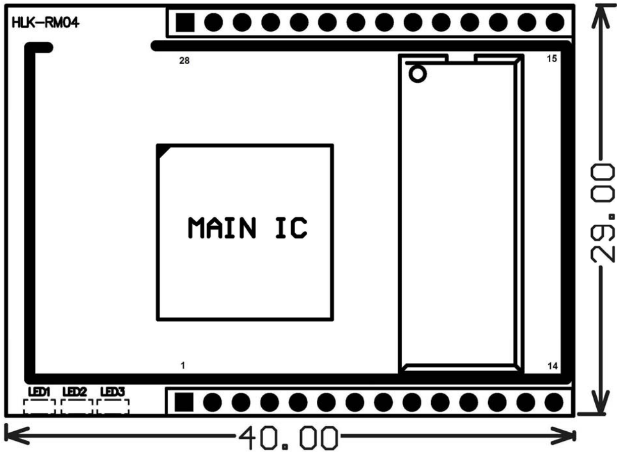
Picture2.Dimensions Unit:mm
