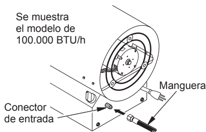
Figura 4: Manguera y conector de entrada
