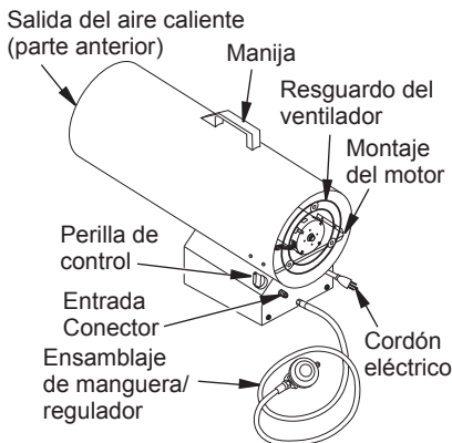
Figura 1: Modelo de 100.000 BTU/h
