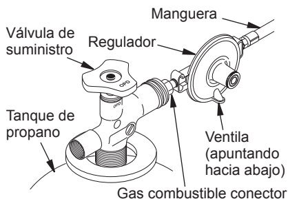
Figura 3: Regulador con ventila apuntando hacia abajo
