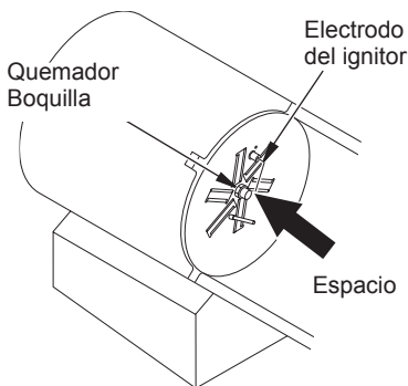
Figura 12: Distancia mínima entre el electrodo del ignitor y la placa de fijación
