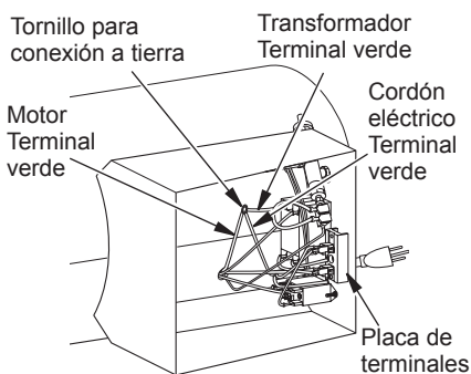
Figura 5: Ubicación del tornillo de conexión a tierra
