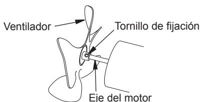
Figura 8: Ubicación del ventilador, del eje del motor y del tornillo de fijación
