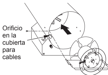
Figura 7: Reemplazo del motor, del montaje del motor y del resguardo del ventilador en el calentador
