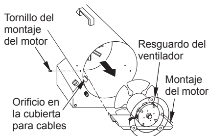
Figura 6: Desmontaje del motor, del montaje del motor y del resguardo del ventilador del calentador
