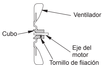
Figura 9: Sección transversal del ventilador
