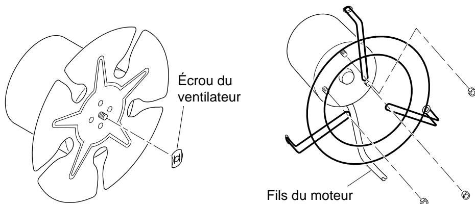
Figure 8 - Retrait de l'écrou du ventilateur de l'arbre du moteur
