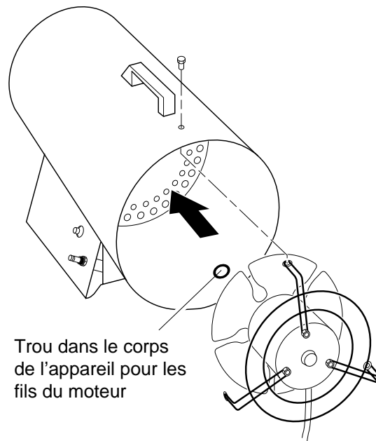
Figure 10 - Remise en place du moteur et de la grille du ventilateur
