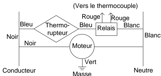
Figure 15 - Schéma électrique en escalier
