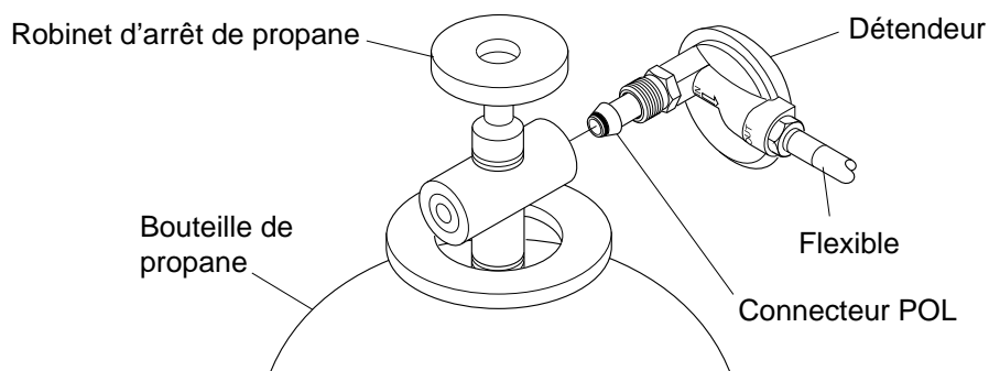
Figure 3 - Positionnement du détendeur
