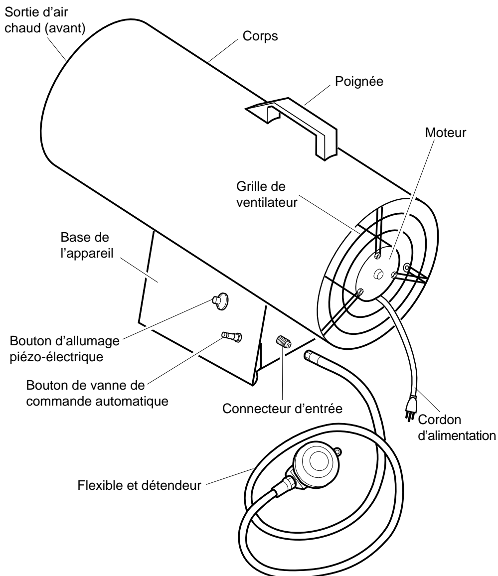
Figure 1 - Modèle 50 000 BTU/hr
