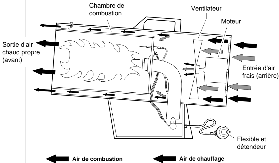
Figure 2 - Vue en coupe de l'appareil en fonctionnement
