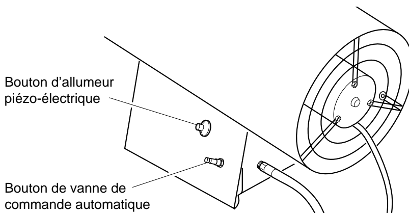
Figure 5 - Boutons de vanne de commande automatique et d'allumeur piézo-électrique
