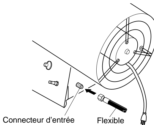
Figure 4 - Flexible et connecteur d'entrée
