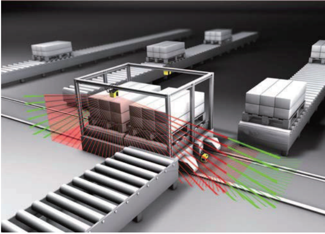
Fig. 4.6-1: Bild 6.3-1 guarding the sides on AGVs
