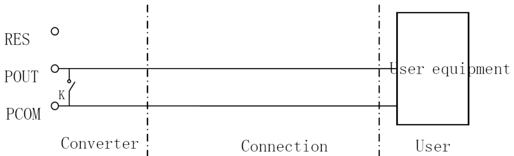
Fig. 8: (c) DS switch connect mode
