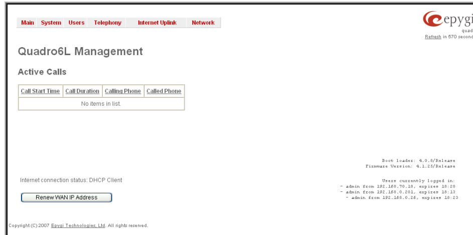
Fig. II-1: Quadro6L Management
