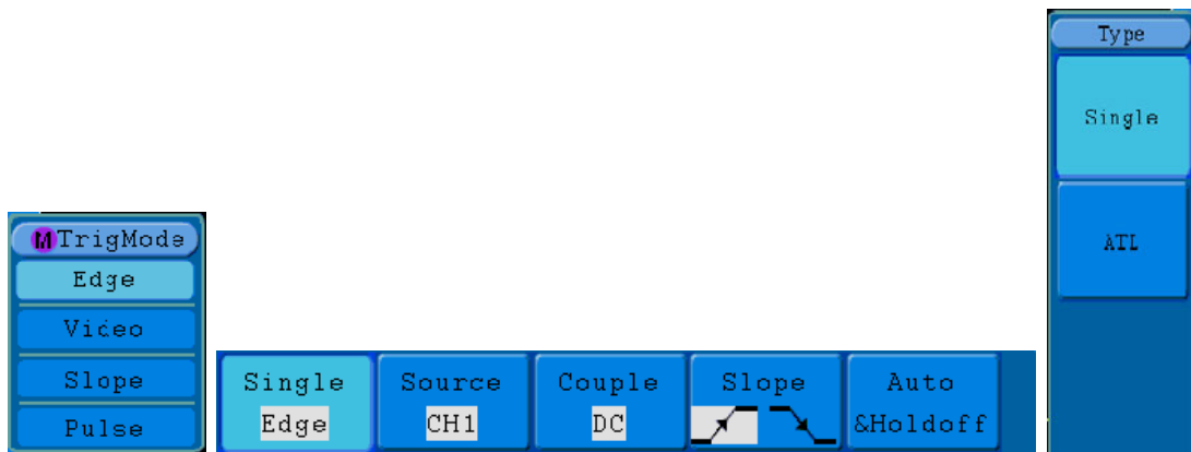
Figure 33. Edge trigger menu.
