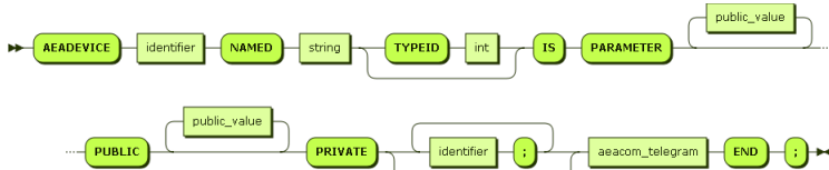
Syntaxgraph 37: aeadevice
