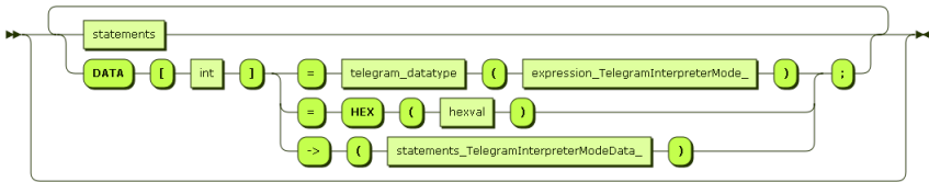
Syntaxgraph 31: telegram_InterpreterMode_
