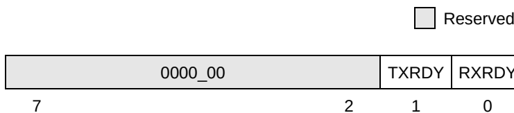
Figure 12-16. DMA Status Register (UDSR)
