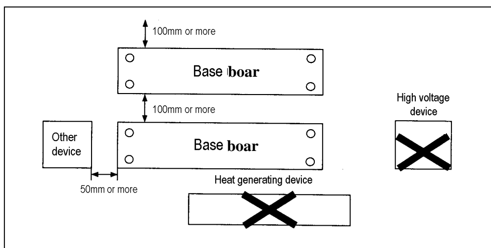
[Fig. 10.1] PLC
