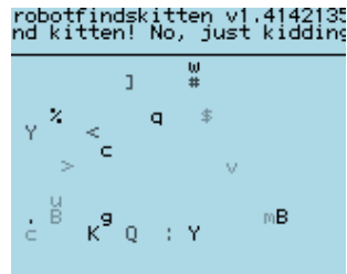
Figure 11.17.: Robotfindskitten
