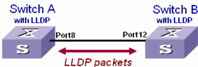
LLDP Example
