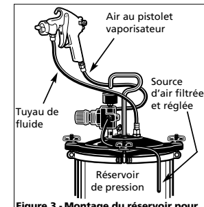
Figure 3 - Montage du réservoir pour l'alimentation sous pression
