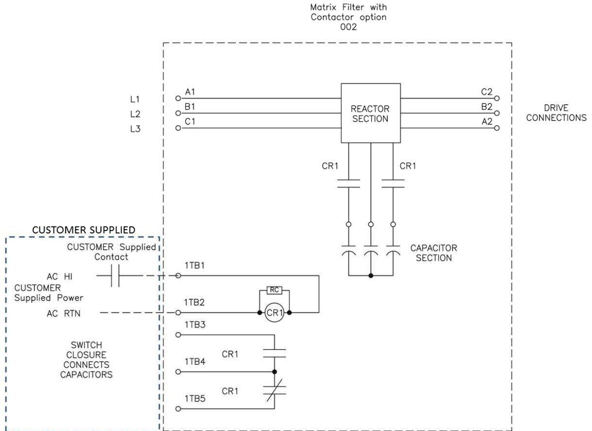
DWG_MNL_0002 Rev. 1
