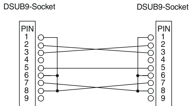
Fig. 3.5: PC data cable DSUB9<>DSUB9
