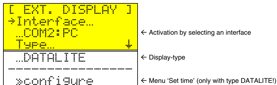
Fig. 5.21: External display 'DATALITE'
