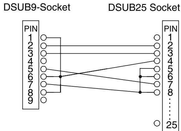
Fig. 3.7: PC data cable DSUB9<>DSUB25
