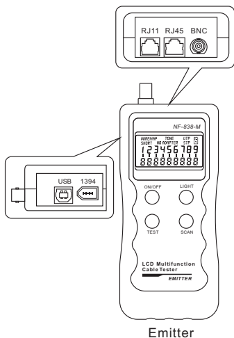
Emitter
