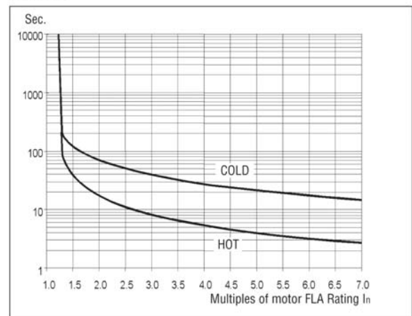
NEMA 20
