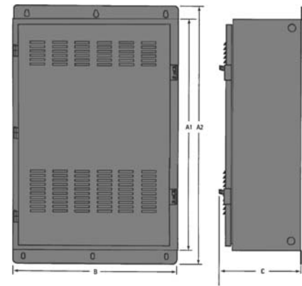
NEMA Type 1
