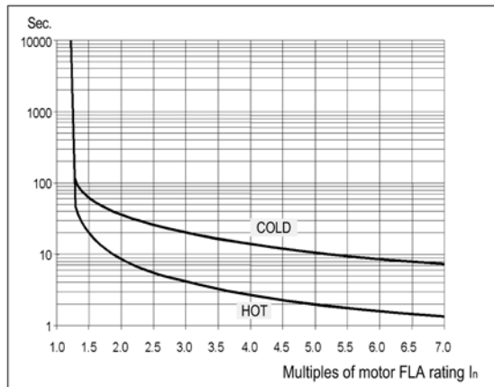
NEMA 30
