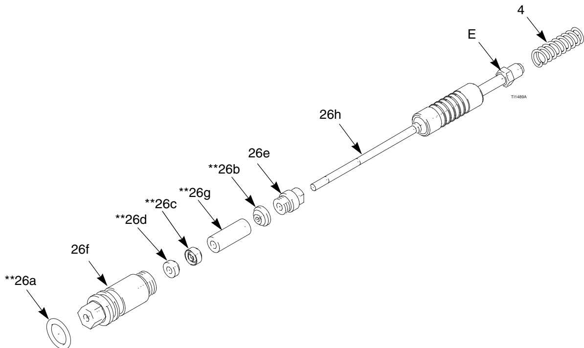
Fig. 27. Packing Rod
