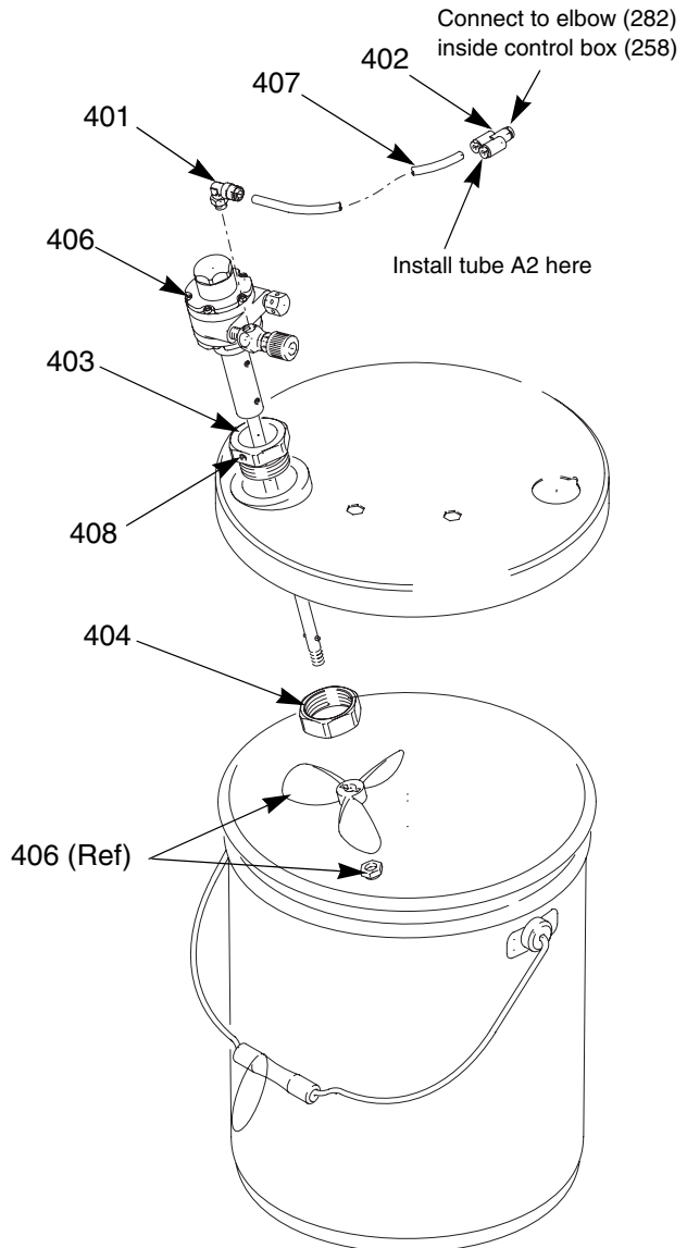
Fig. 11. 245895 Agitator Kit
