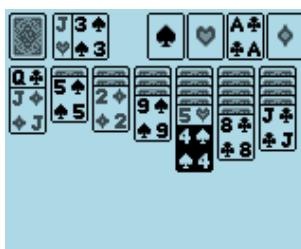
Figure 11.22.: Klondike solitaire
