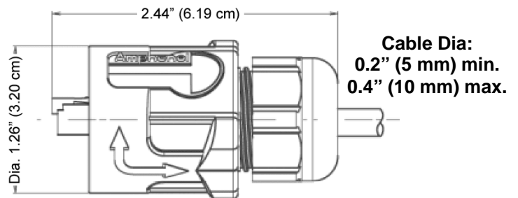
ET-RJFRB-6 (IP67 Ethernet Plug)
