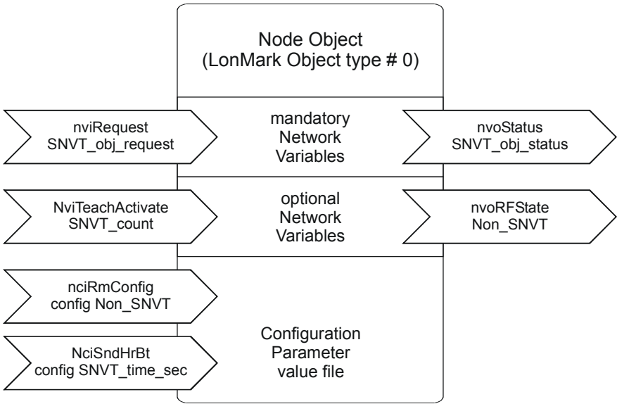
Fig. 15. Node Object
