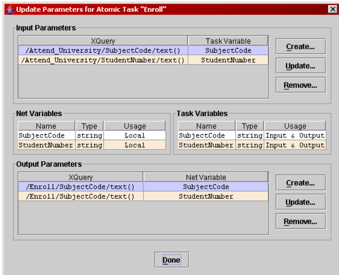
Fig. 33. Established task parameters
