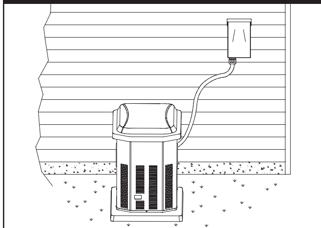
Figure 54 — Assemblage Typique d'un Boîtier de Débranchement
