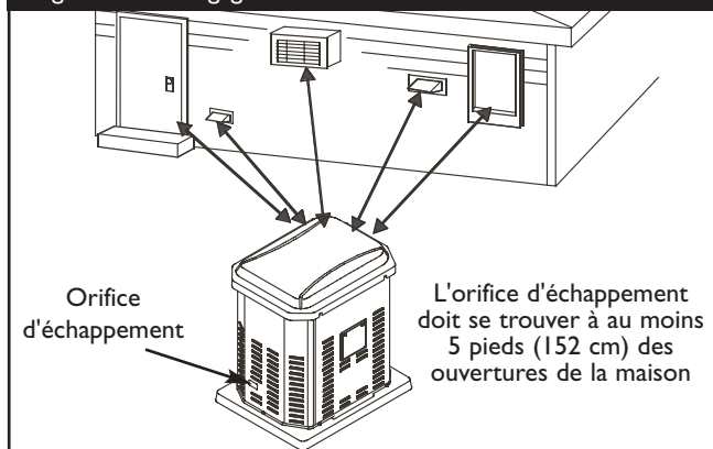
Figure 52 — Dégagement du Génératrice d'état d'attente
