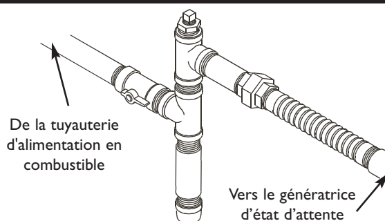
Figure 57 — Raccords de Combustible Complétés
