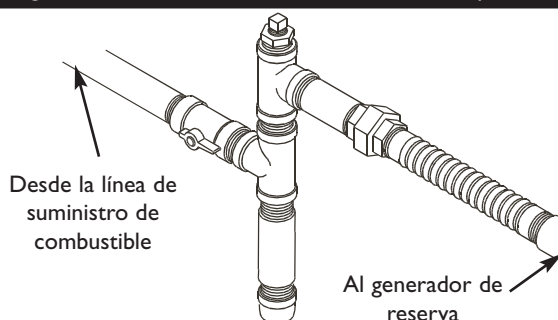
Figura 44 — Conexiones de Combustible Completas
