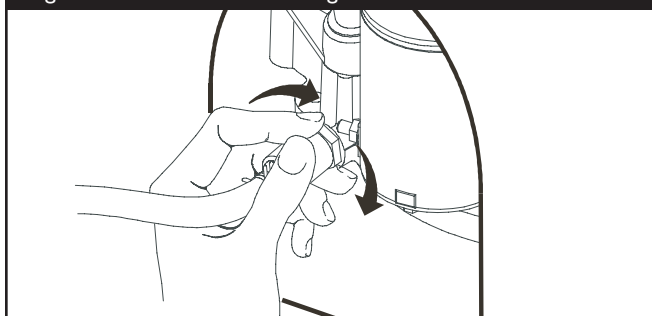
Figure 63 — Raccord de Vidange d'Huile
