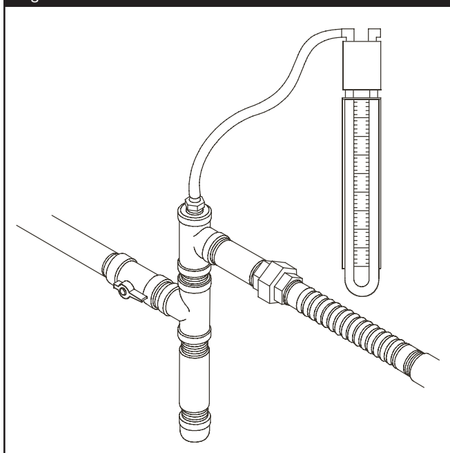
Figura 43 — Manómetro Instalado Transitoriamente
