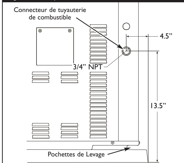
Figure 55 — Emplacement du Combustible et des Éléments
