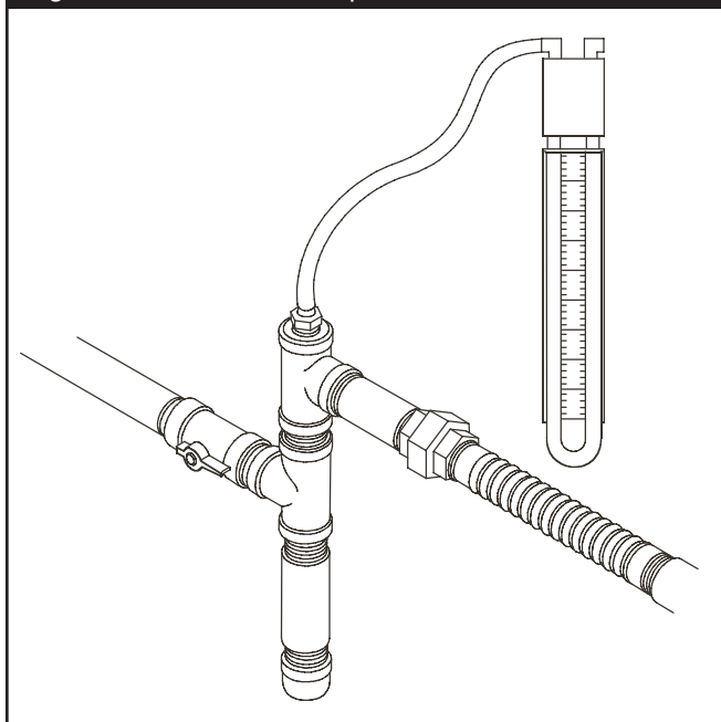
Figure 56 — Manomètre Temporaire Installé
