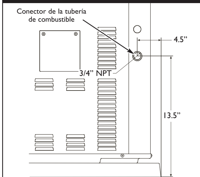
Figura 42 — Ubicación de los Accesorios del Combustible del Generador
