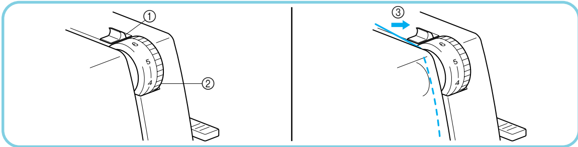
① Botón de liberación de la tensión del hilo ② Disco de tensión del hilo ③ Deslízcela hacia la derecha.
