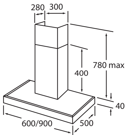
T-CANOPY
