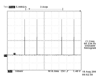
2 U501-#44 V-SYNC
