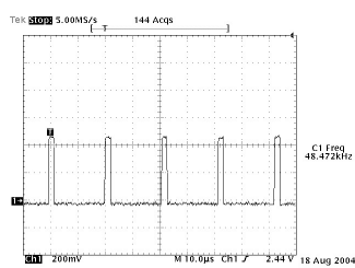
2 U501-#43 H-SYNC
