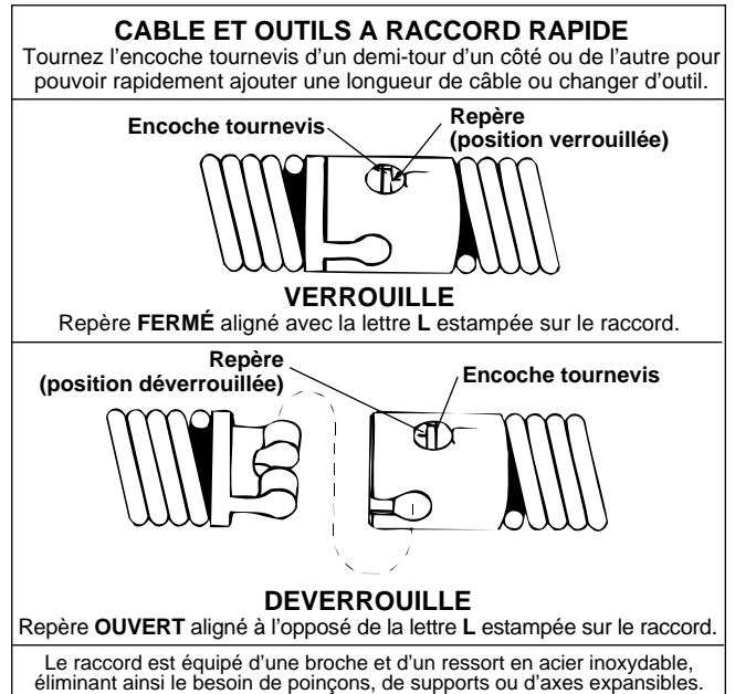
Figure 3 – Accouplement/désaccouplement d'un câble et d'un raccord flexible ou outil
