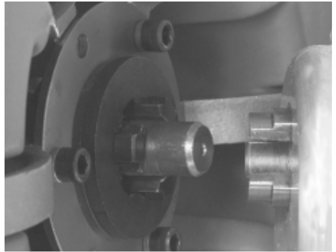
Figura 12 – Instalación del conjunto del tambor hacia la caja de engranajes
