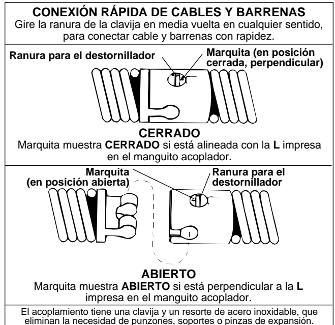
Figura 3 – Conexión/desconexión del cable a la colita de cerdo o a diversas barrenas
