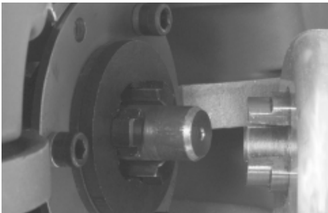
Figure 12 – Montage du tambour sur le boîtier
