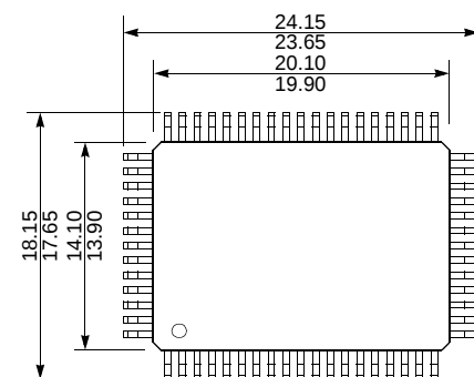
64MQFP
