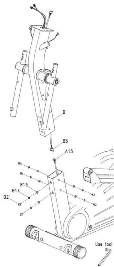
ABB. 4- Montieren des Computers
