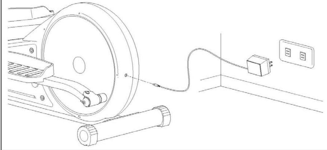
ABB. 9- Anbringen des Adapters
