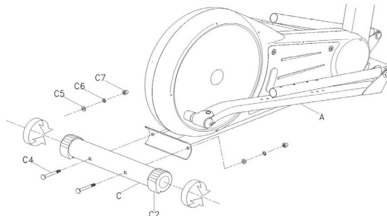
ABB. 1- Montieren der hinteren Querstütze
