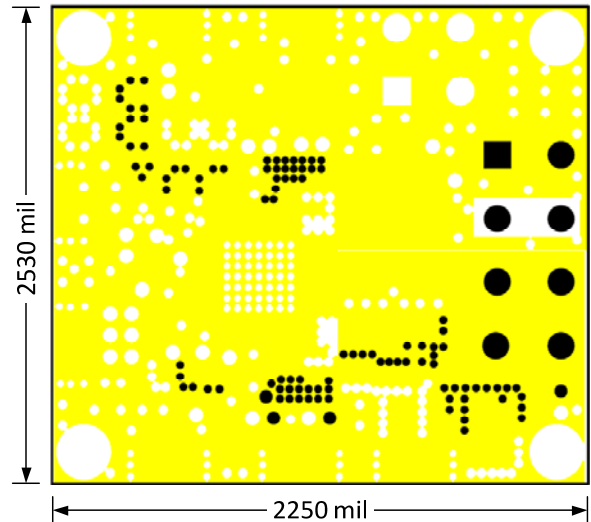
Mid Layer 2
