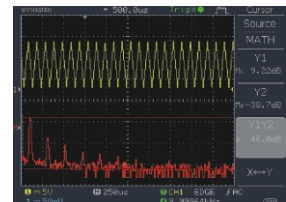
FFT Function
