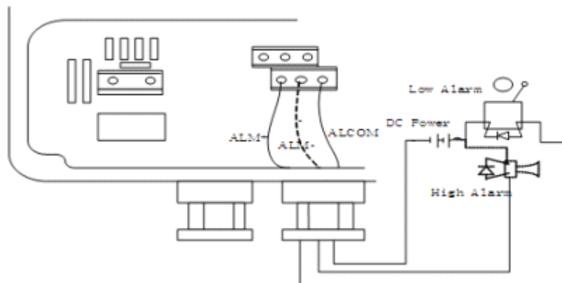
Fig. 14(d) Digital Output Direct Connection
