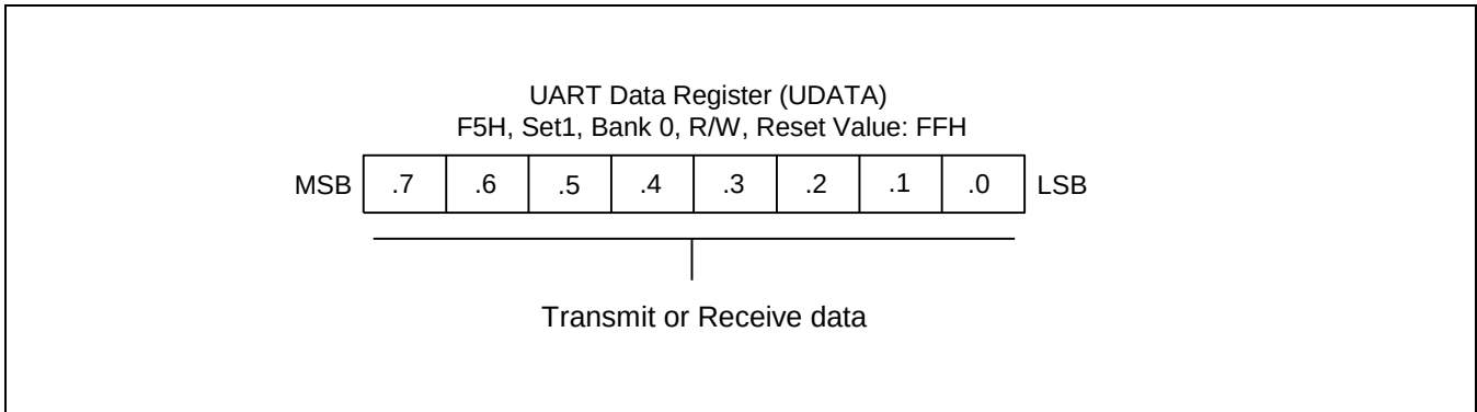
Figure 15-3 UART Data Register (UDATA)
