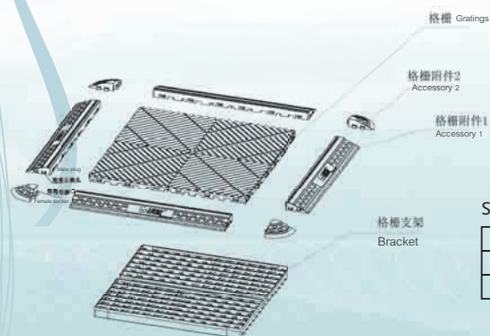
正面 部件爆炸图
