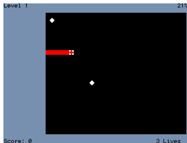
Figure 11.30.: Xobox
