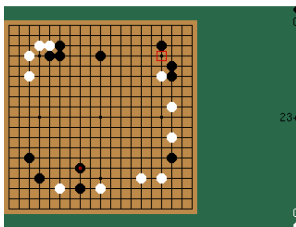
Figure 11.10.: Goban
