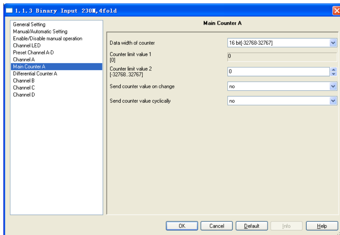
Fig.5.14 (2) Parameter window “Main Counter X”
