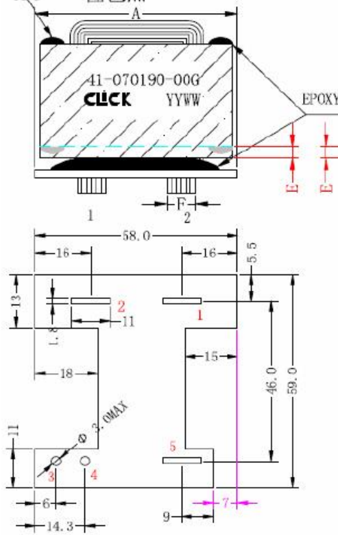
顶视图
