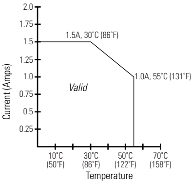
FET Current per Point (1762-L24BXB, L40BXB 1762-L24BXR, L40BXR)
