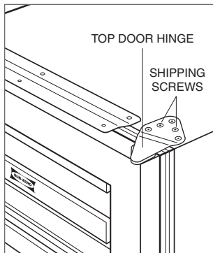
Top hinge.
