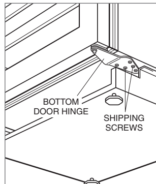
Bottom hinge.
