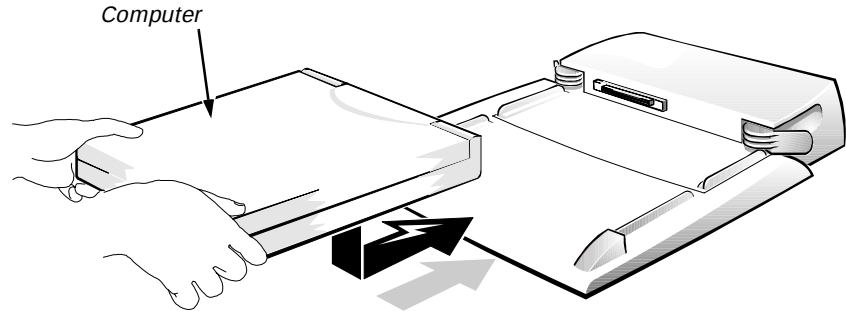
Abbildung 3-2. Computer auf den Port Replicator platzieren
