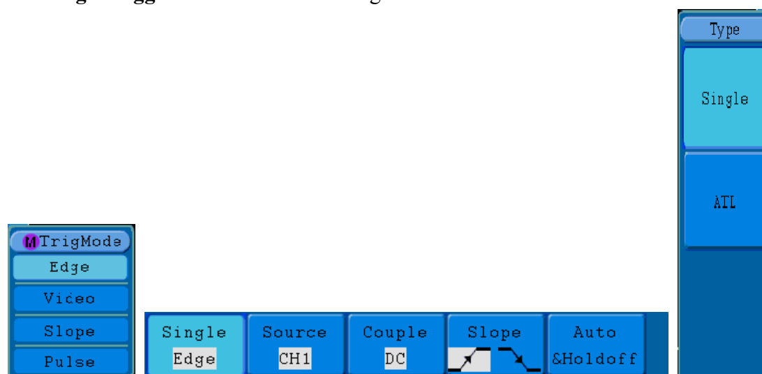
Fig. 5-17 Edge trigger menu
