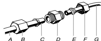
A. Tubería de agua del refrigerador B. Tuerca (provista) C. Bulbo D. Acoplamiento (adquirido) E. Férula (adquirida) F. Tuerca (adquirida) G. Línea de agua de la casa
